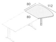
ART. WM 418 DX - SX ANGOLO ASIMMETRICO 90°
